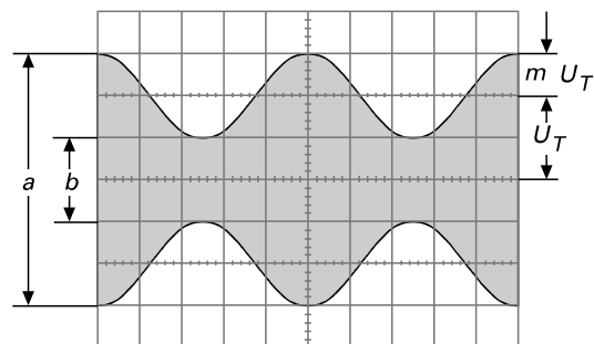
Figure 2 Ondulation modulée en amplitude : F = 1MHz ; f = 1kHz ; m = 50% ; UT = 28,3mV eff . En relevant les deux valeurs a et b sur l'écran, le taux de modulation se calcule par
